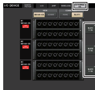
VIRTUAL RACK 画面 (EXTERNAL HA ページ)
