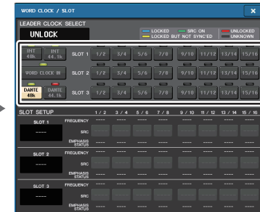
WORD CLOCK/SLOT SETUP 画面
